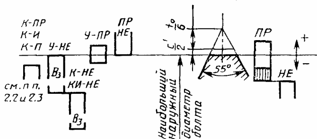
Калибры для контроля болтов (наружной резьбы)
