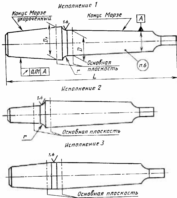
Размеры, мм
