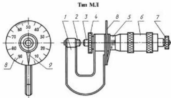
1 — скоба; 2 — гайка; 3 — микрометрический винт; 4 — стопор; 5 — стержень; 6 — барабан; 7 — трещотка (фрикцион); 8 — штифт; 9 — стрелка
