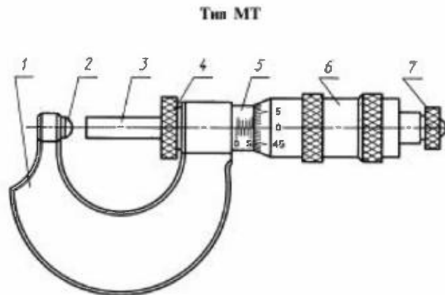
1 — скоба; 2 — гайка; 3 — микрометрический винт; 4 — стопор; 5 — стержень; 6 — барабан; 7 — трещотка (фрикцион)
