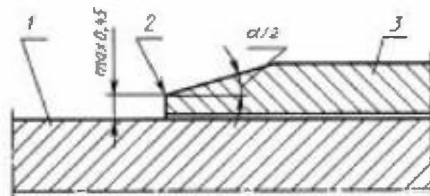
1 — поверхность стебля; 2 — измерительная кромка; 3 — барабан
