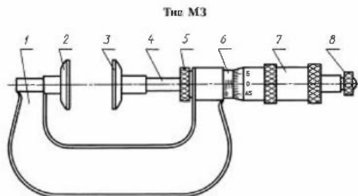
1 — скоба; 2 — гайка; 3 — измерительная губка; 4 — микрометрический винт; 5 — стержень; 6 — барабан; 7 — трещотка (фрикцион); 8 — трещотка (фрикцион)
